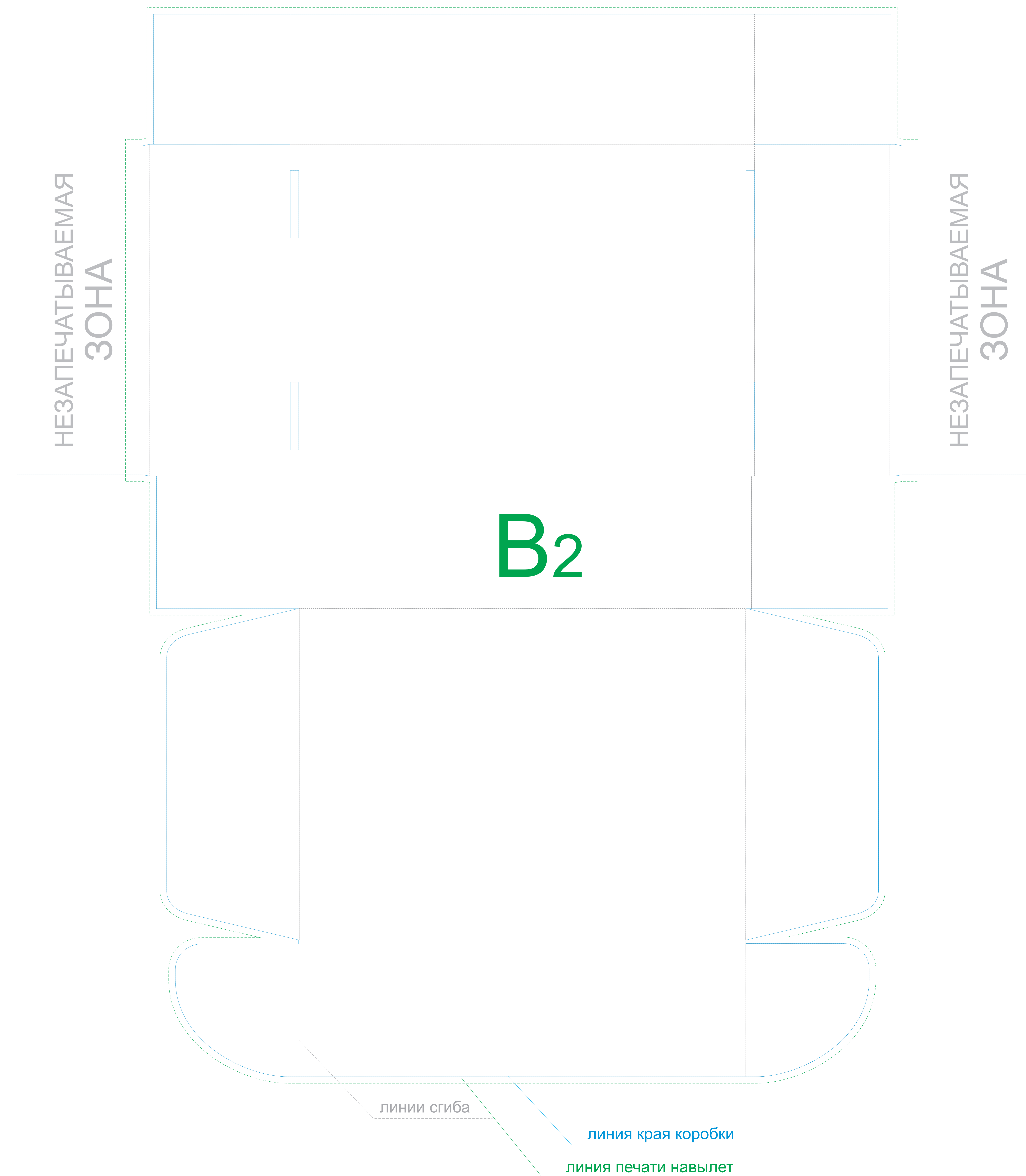
Коробка в разложенном виде ВНУТРЕННЯЯ СТОРОНА
