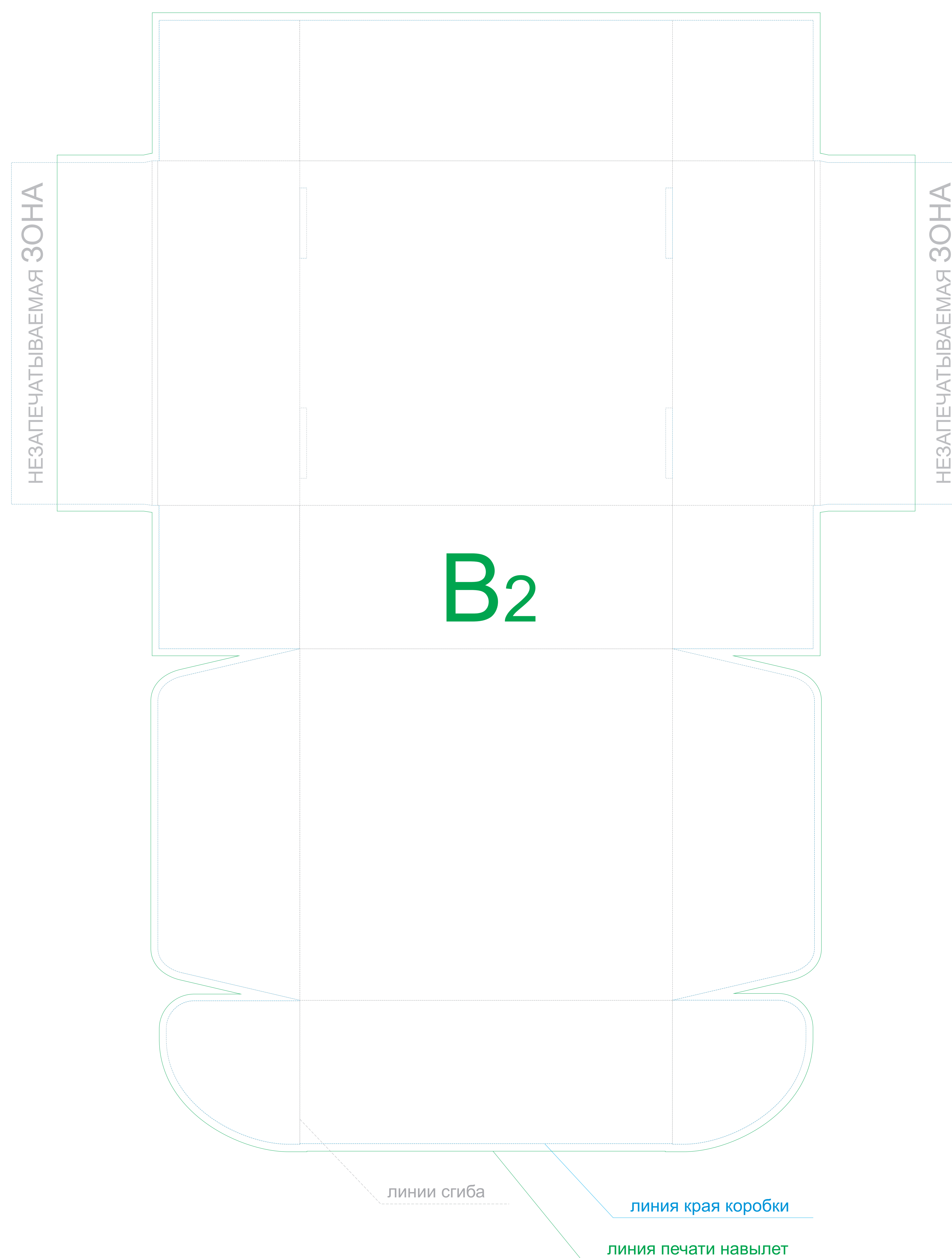
Коробка в разложенном виде ВНУТРЕННЯЯ СТОРОНА
